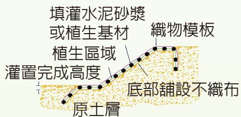
剖面圖
